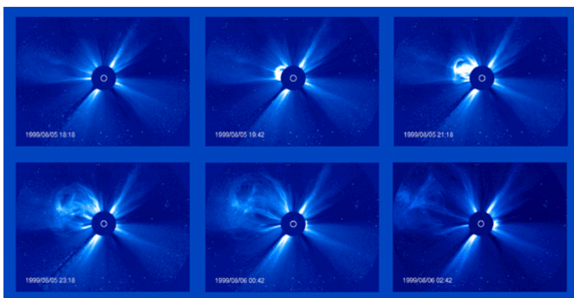
Figura 15: Sequência de imagens de coronógrafo mostrando uma CME, desde o momento da formação até o completo desprendimento da coroa solar. Fonte: http://sohowww.nascom.nasa.gov/gallery/images/large/cmeprogchart_prev.jpg
