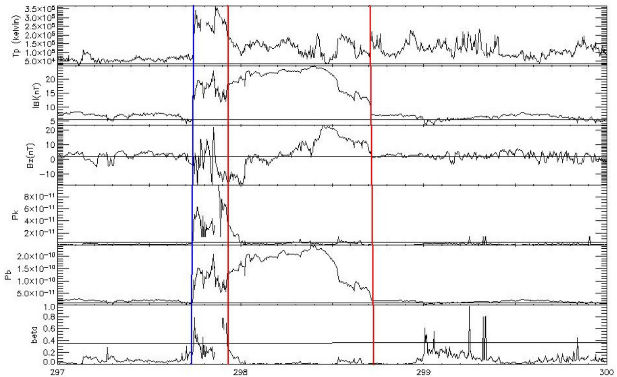
Figura 36: Paineis com os gráficos do meio interplanetário de Outubro de 2011.
