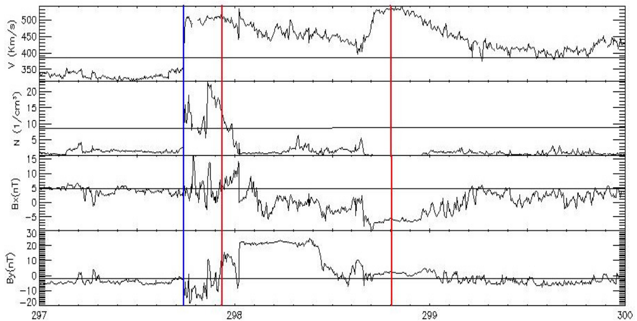
Figura 37: Painel mostrando os gráficos dos demais parâmetros interplanetários para Outubro de 2011.
