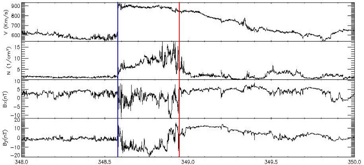
Figura 34: Painel mostrando gráficos dos demais parâmetros interplanetários analisados para Dezembro de 2006.
