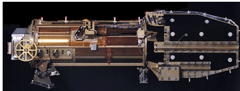
Figura 29: Imagem do telescópio EIT. Fonte: http://umbra.nascom.nasa.gov/eit
