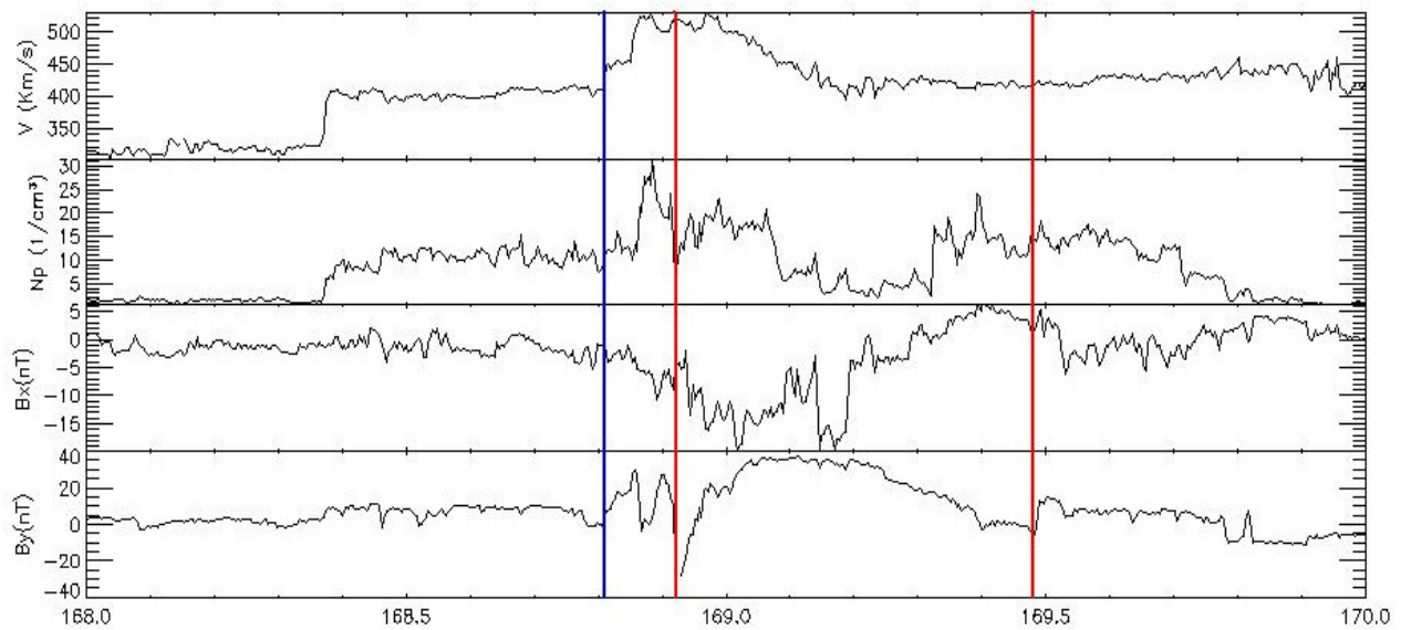
Figura 39: Painel mostrando os gráficos dos demais parâmetros interplanetários de junho de 2012.
