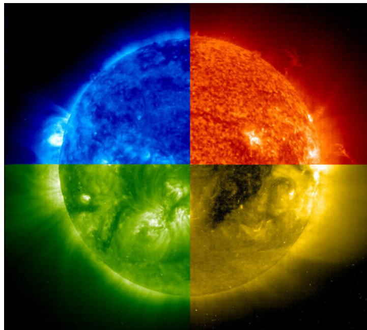
Figura 28: O Sol dividido em quatro quadrantes, onde cada quadrante corresponde a um comprimento de onda distinto. Fonte: http://sohowww.nascom.nasa.gov .
