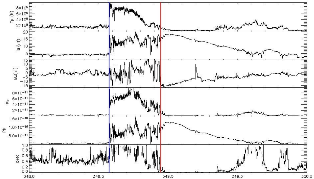
Figura 33: Paineis com os gráficos do meio interplanetário de Dezembro de 2006.
