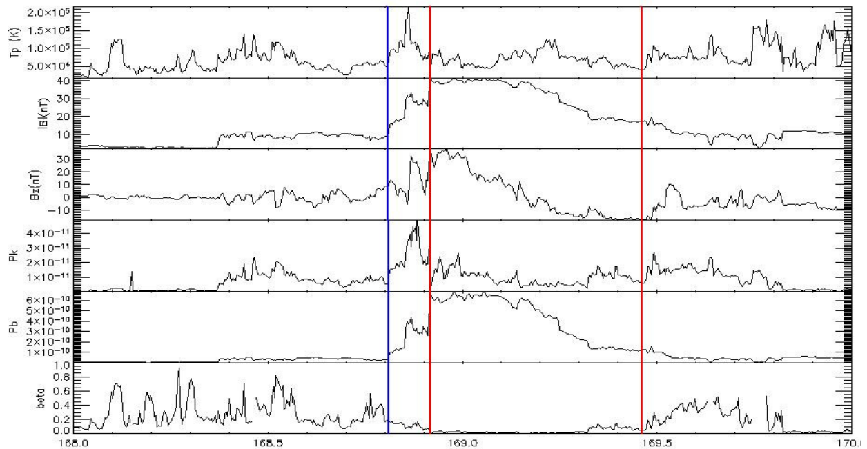
Figura 38: Painele mostrando os gráficos do meio interplanetário de junho de 2012.
