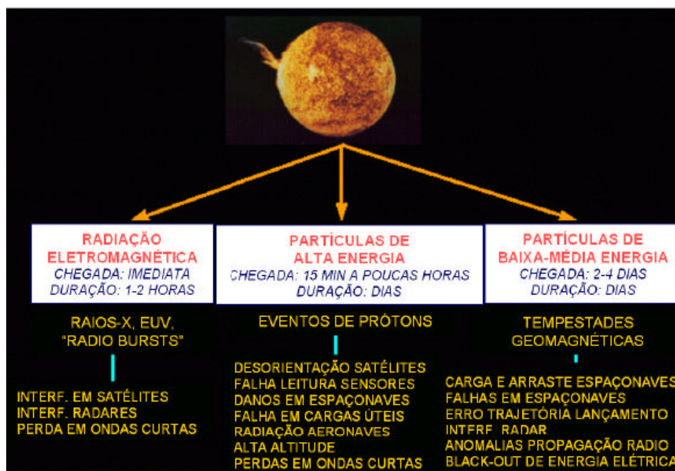
Figura 23: Fenômenos que afetam o Clima Espacial, energias envolvidas, tempo de duração de seus efeitos e principais tipos de danos em sistemas tecnológicos. Fonte: Schwenn (comunicação pessoal), (apud Dal Lago, 2003).
