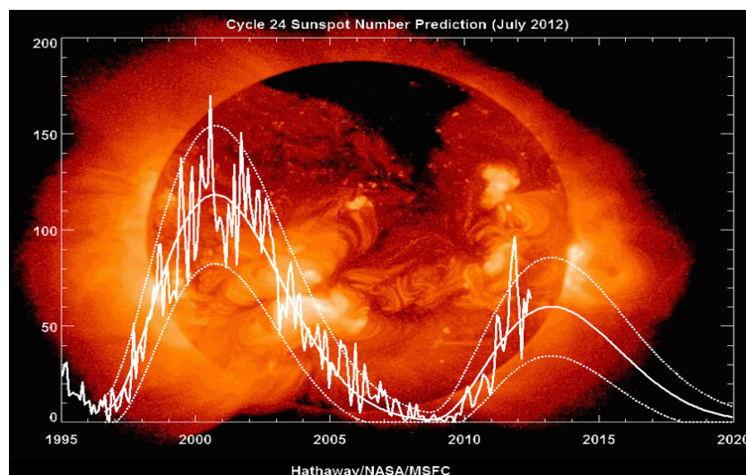
Figura 10: Previsão para o próximo máximo solar
