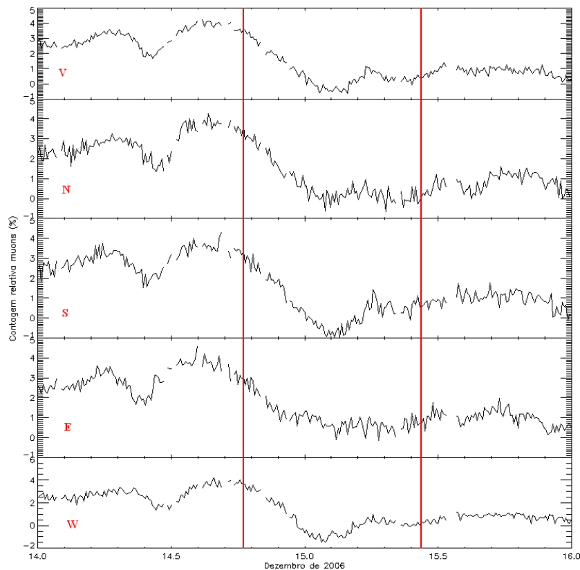
Figura 35: Contagem relativa de muons nas direções vertical (V), norte 30° (N), sul 30° (S), leste 30° (E) e oeste 30° (W), mostrando o decréscimo de Fourbush relacionado a uma tempestade geomagnética.
